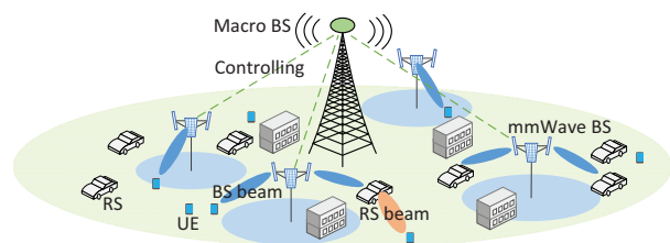
Fig. 1. Network scenario.
